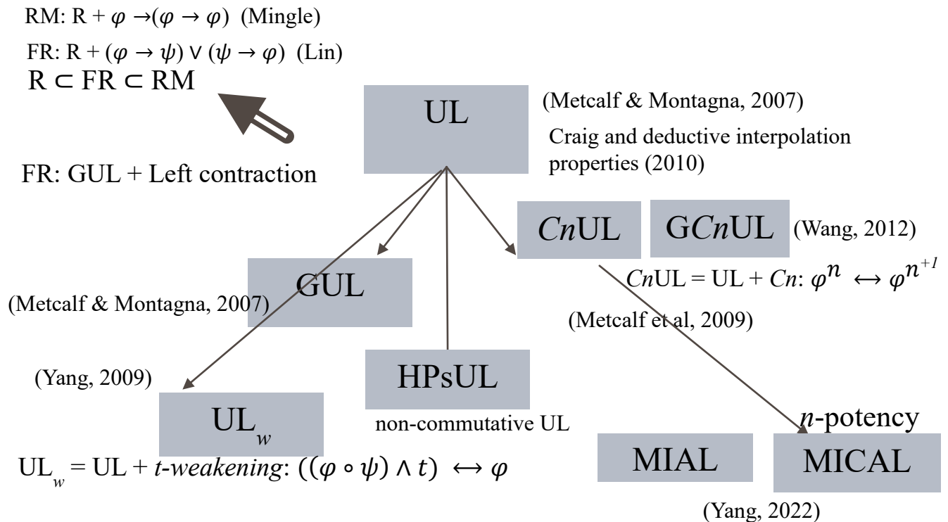
شکل ۱. نمودار توسعه‌ی منطق‌های فازی ربطی توسعه UL و RM
